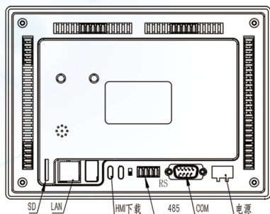
背视图
