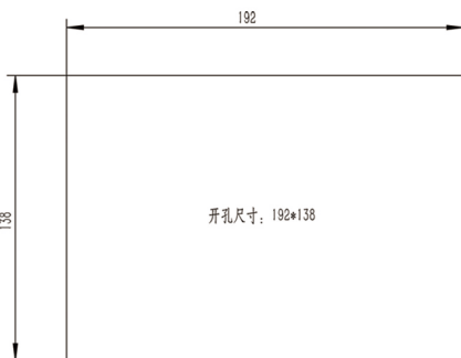
开孔尺寸图
